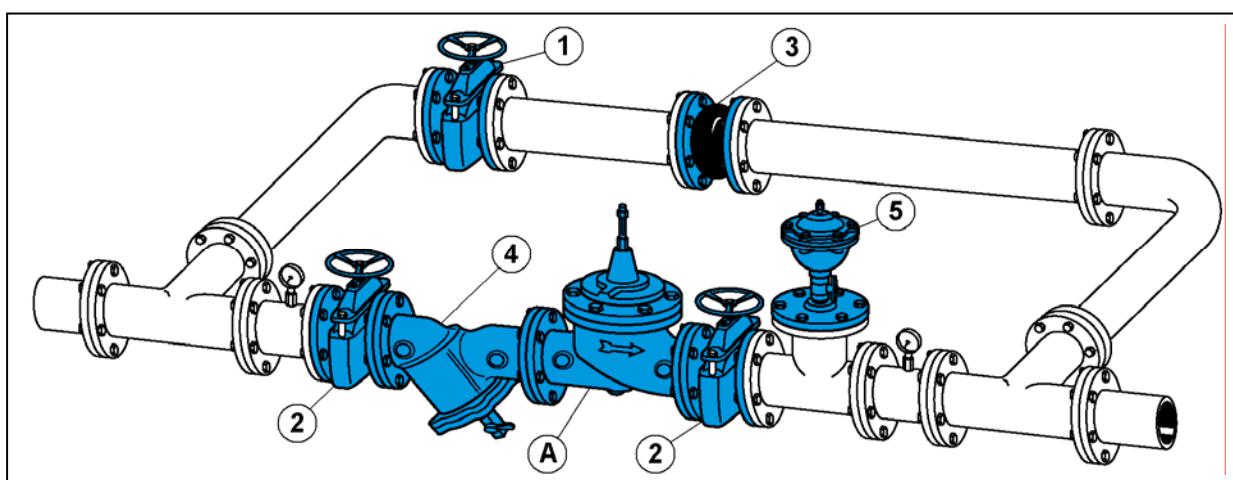
Рис. 1 Пример установки регулятора давления S101.
