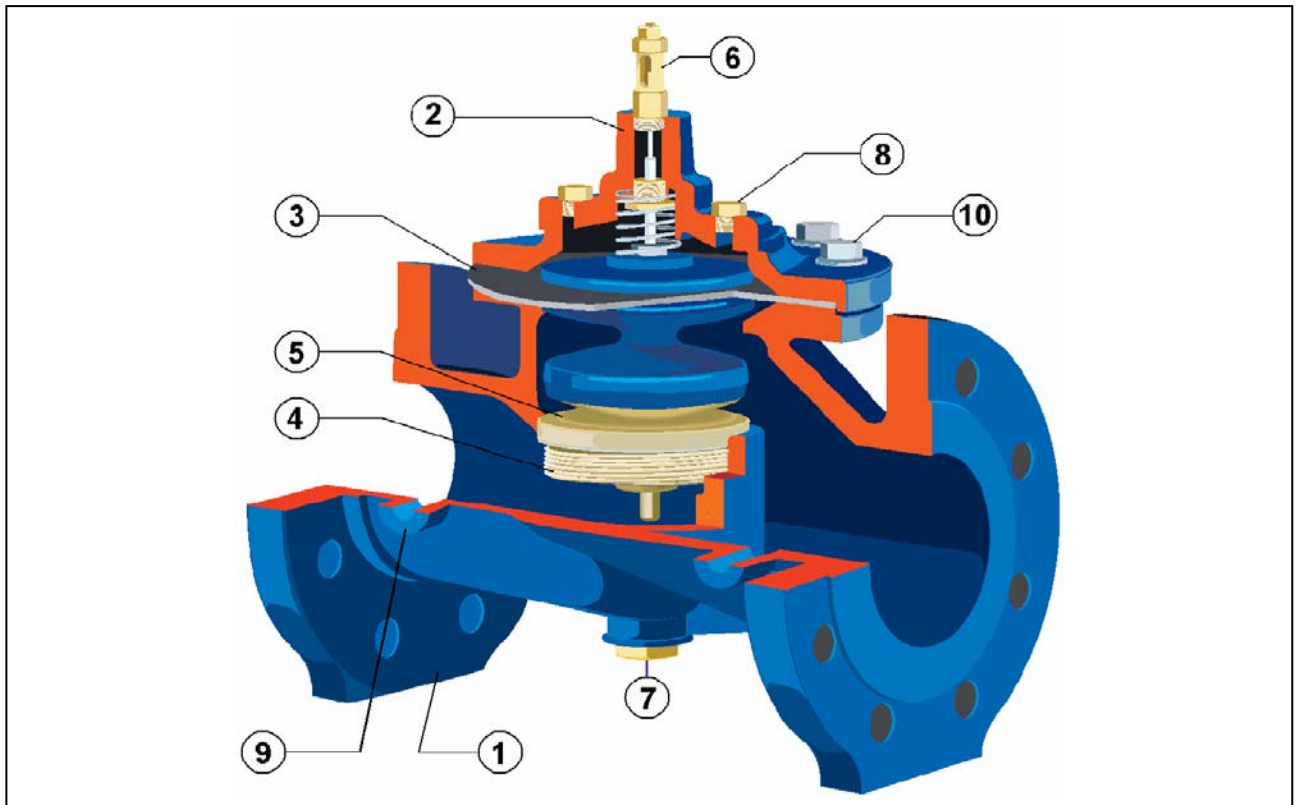
Рис. 1 Устройство основного клапана.
