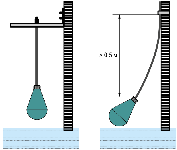
1) 2) Рисунок 3.1 – Монтаж на объекте
