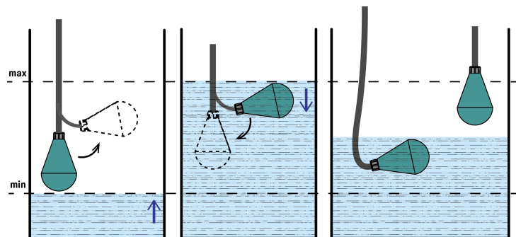
1) 2) 3) Рисунок 4.2 – Принцип действия
