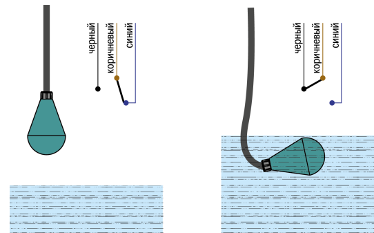
1) 2) Рисунок 4.1 – Переключение ПСУ
