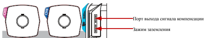
Рис. 0-6 Использование сигнала компенсации
