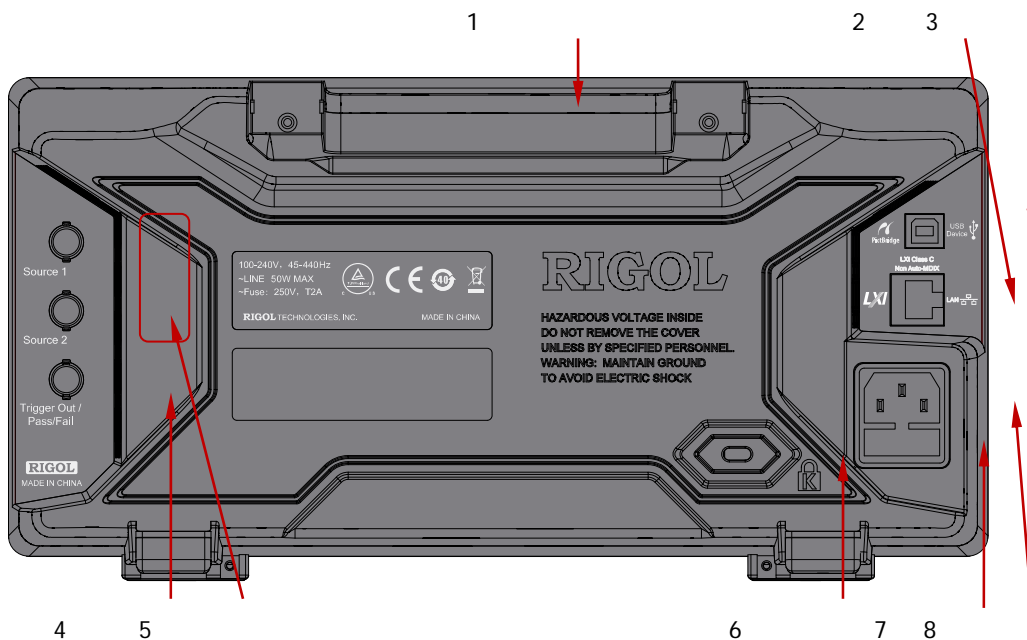
Рис. 0-10 Общий обзор задней панели.
